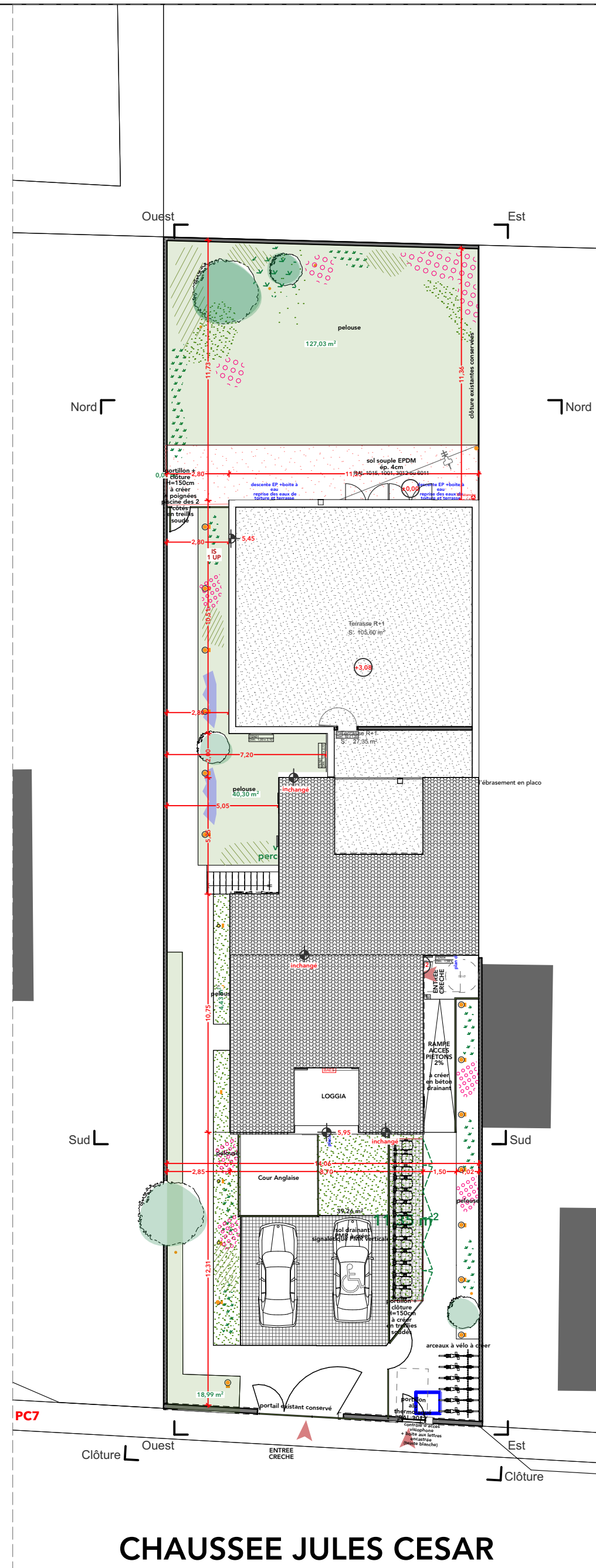
Plan masse - Projet
